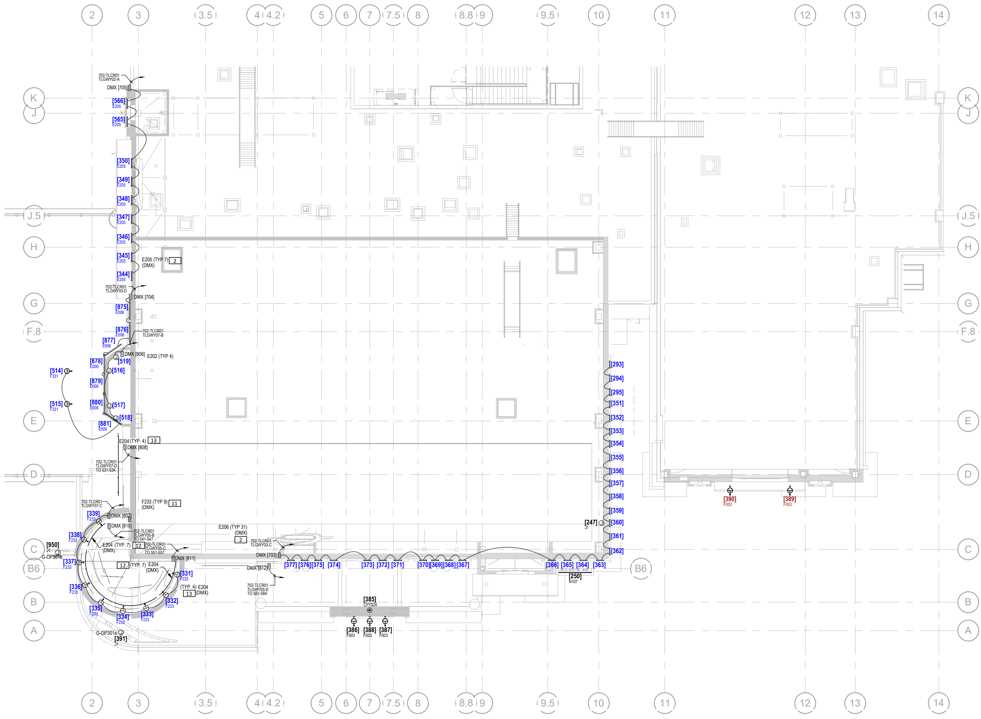
外立面平面图 - 主题灯光 1 EXTERIOR - FACADE PLAN - THEMED LIGHTING TL201
